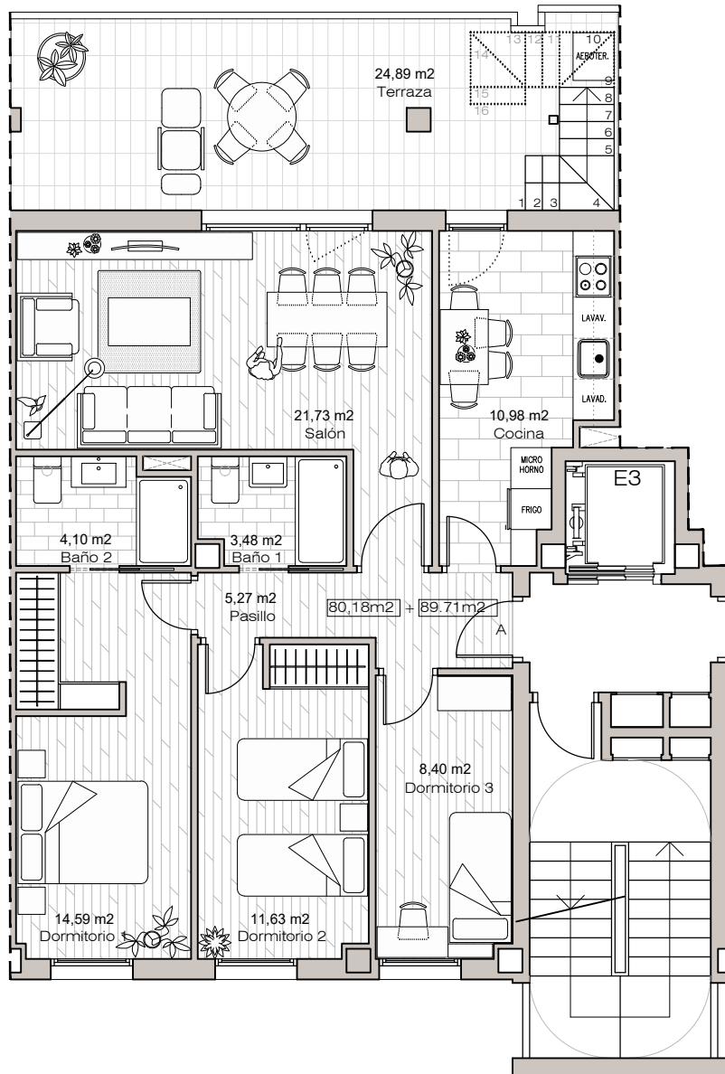
PLANTA OCTAVA
